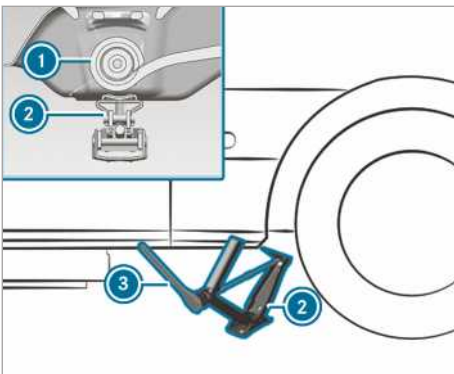
Място за поставяне на крик, заден мост
