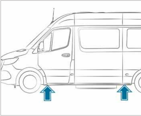
Места за поставяне на крика
