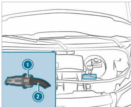
OM651 achterwielaandrijving
