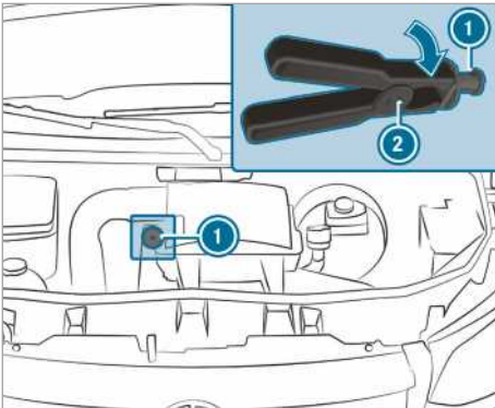
Käynnistysapuvirtapiste (esimerkki)
