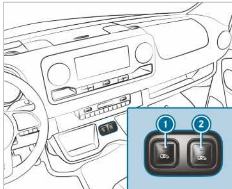
Keskikonsolin liukuovinäppäin
