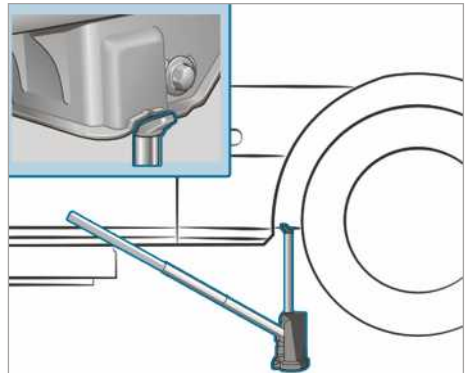
Autóemelő felfekvési pontja, hátsó tengely (5,0 tonnás gépkocsik)
