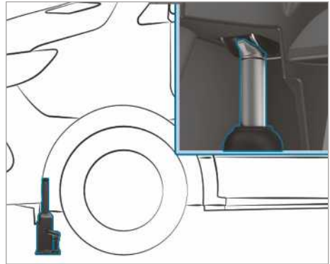
Kriksteunpunt, vooras
