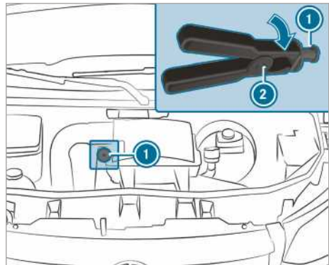
Hulpstartpunt (voorbeeld)
