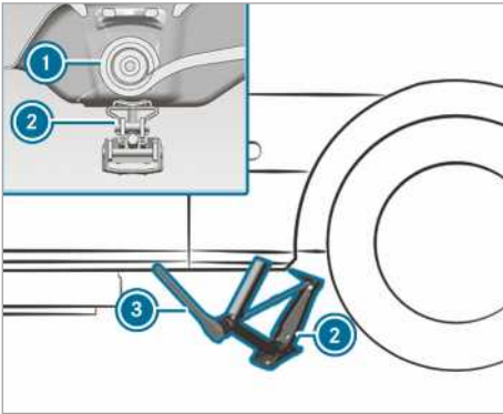
Приемная точка для автомобильного домкрата, задний мост
