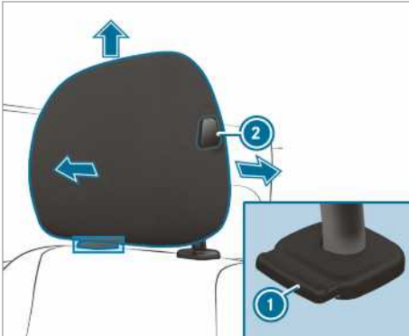
Hoofdsteun (voorbeeld comforthoofdsteun op chauffeursstoel)
