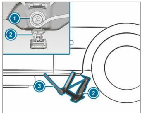
Място за поставяне на крик, заден мост
