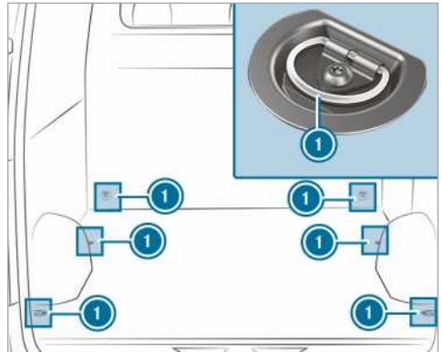
Точки за прикрепване (пример фургон без носещи шини)
