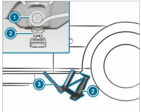
Kriksteunpunt, achteras
