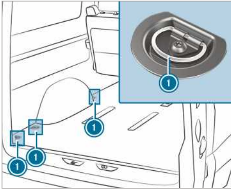
Points d'arrimage (exemple: combi)
