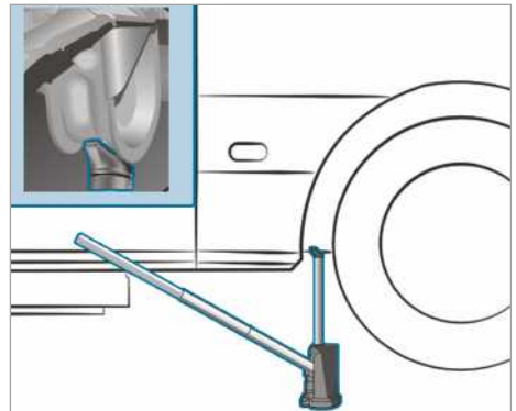
Point d'appui du cric, essieu arrière (exemple: fourgon et combi jusqu'à 4,0 t)
