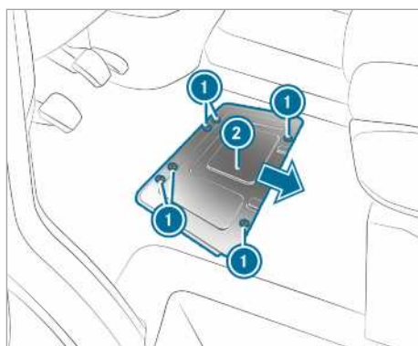
Véhicules à traction avant
