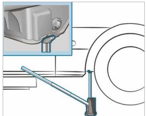
Point d'appui du cric, essieu arrière (véhicules 5,0 t)
